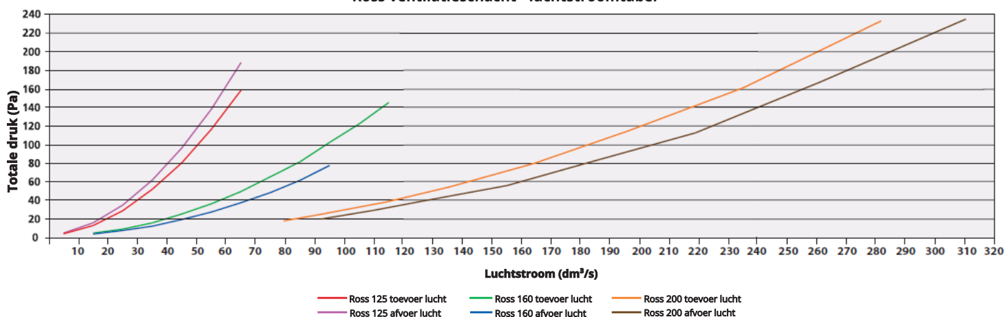
Ross ventilatieschacht - luchtstroomtabel
